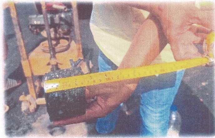
รูปภาพ ; โครงการซ่อมแซมถนน คสล. โดยวิธีเททับด้วยยางแอสฟัลท์ติกคอนกรีต ถนนสายจากหมู่บ้านไปวัดป่าเวฬุวัน ม.9 บ.หินโงม
