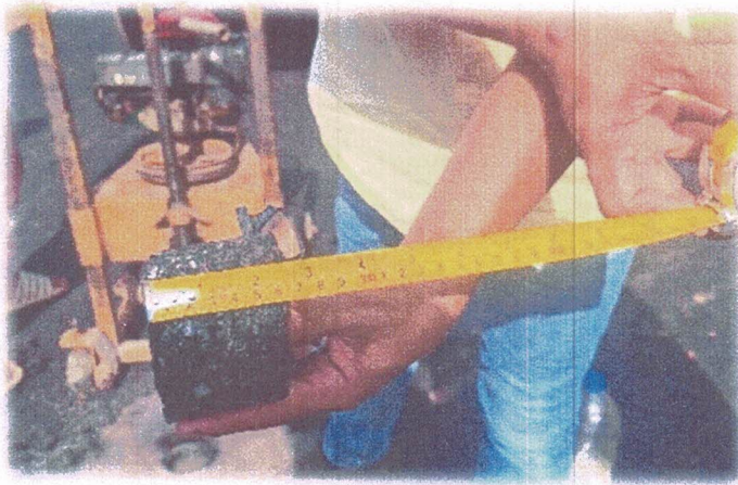
รูปภาพ ; โครงการซ่อมแซมถนน คสล. โดยวิธีเททับด้วยยางแอสฟัลต์ติกคอนกรีต ถนนสายจากหมู่บ้านไปวัดป่าเวสุวัน ม.9 บ.หินโงม
