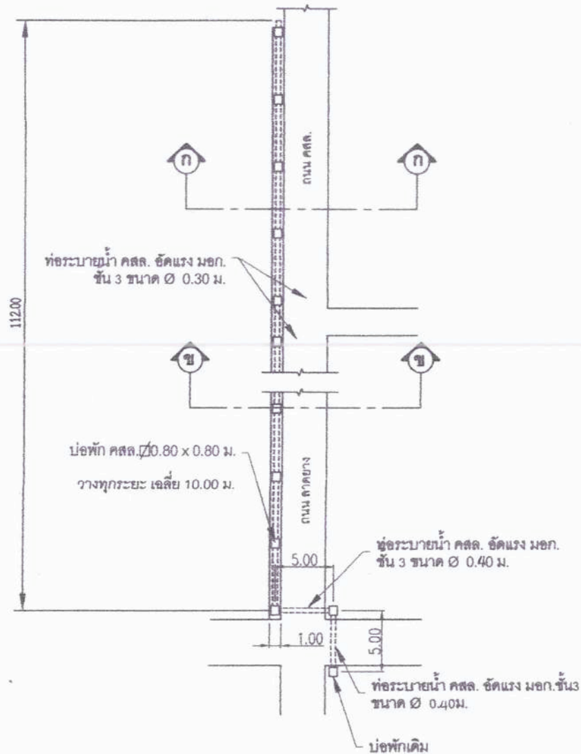
แปลนวางท่อและรางวี NOT TO SCALE
