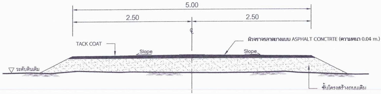
รูปตัดโครงสร้างทางแบบ ASPHALT CONCRETE NOT TO SCALE
