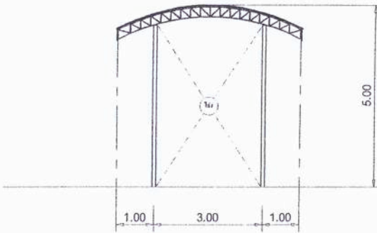
รูปด้านหน้าจุดปรับปรุง 2
