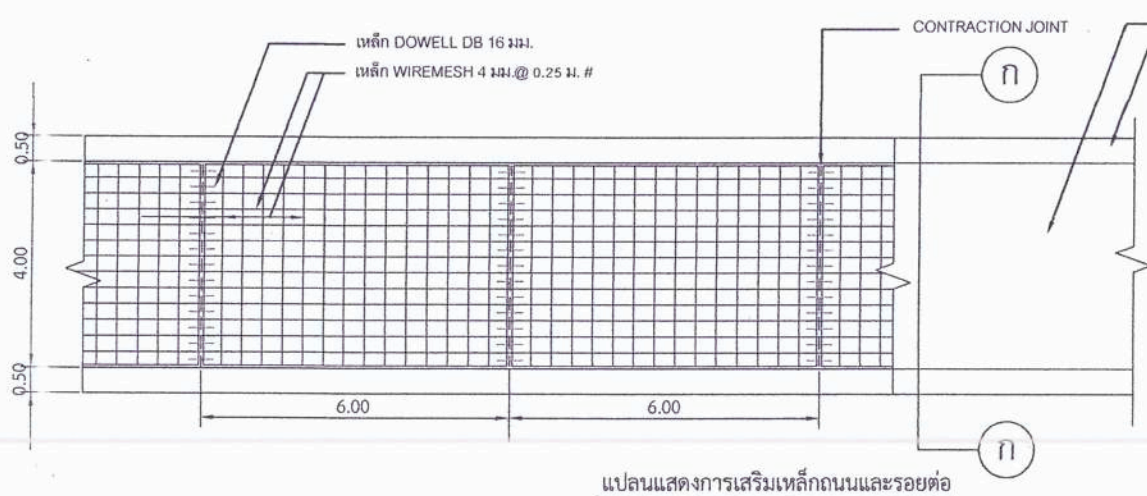
แปลนแสดงการเสริมเหล็กถนนและรอยต่อ
