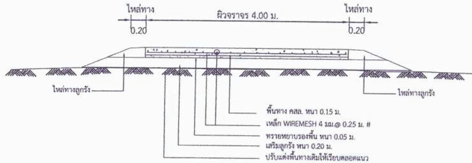
รูปตัดถนน ก - ก
