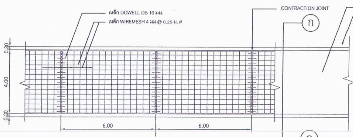
แปลนแสดงการเสริมเหล็กถนนและรอยต่อ
