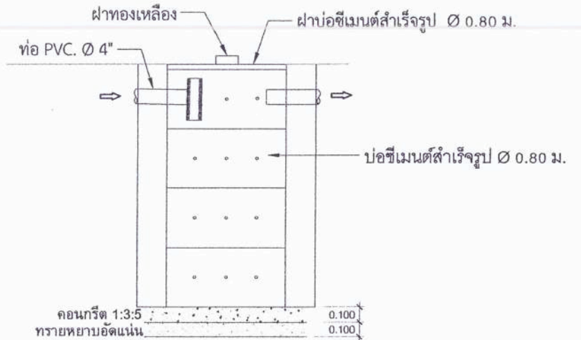
รูปตัดบ่อรับน้ำเสีย
