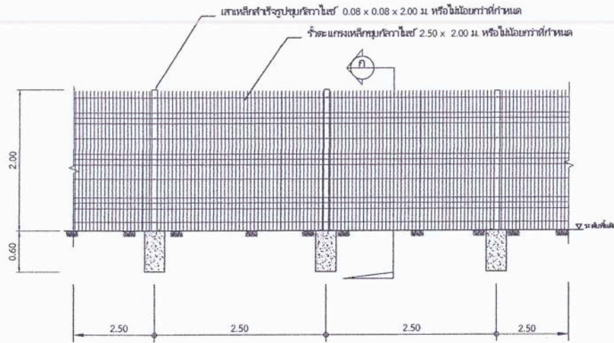
รูปด้านรี NOT TO SCALE
