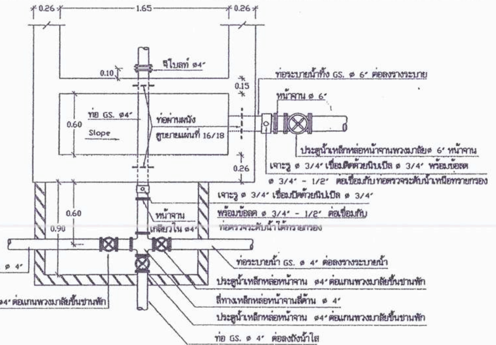
แบบขยายการประสานท่อออกจากถังกรอง 1 : 25
