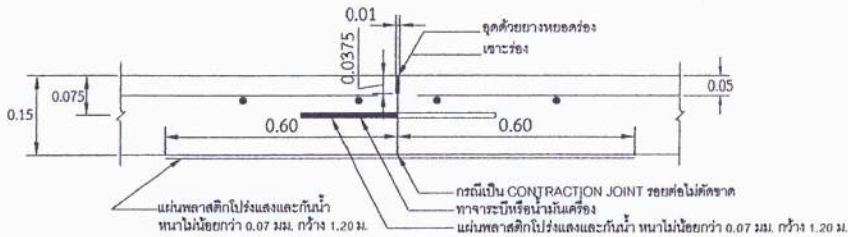
ขยายรอยต่อ CONTRACTION JOINT และ CONSTRUCTION JOINT
