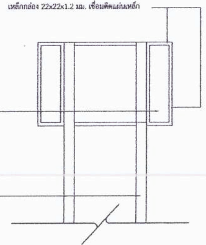
รูปด้านหลังแบบป้ายภายหลังการก่อสร้างเสร็จ มาตราส่วน 1:25
