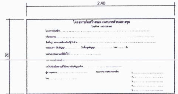
รูปด้านหน้าแบบปายระหว่างการก่อสร้าง มาตราส่วน 1:25
