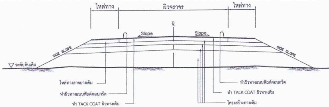
รูปตัดโครงสร้างทาง 2 NOT TO SCALE
