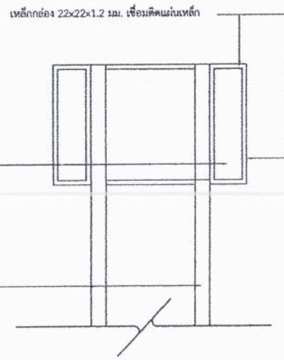
รูปด้านหลังแบบป้ายภายหลังการก่อสร้างเสร็จ มาตราส่วน 1:25
