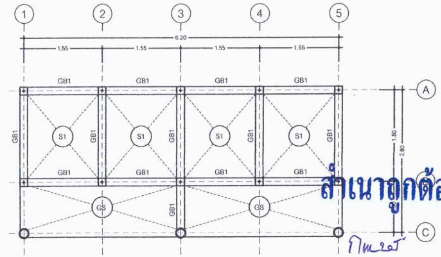
แปลนคานาคอดิน/พื้น มาตราส่วน 1:50
