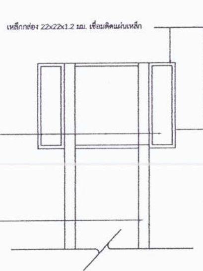
รูปด้านหลังแบบปายภายหลังการก่อสร้างเสร็จ มาตราส่วน 1:25
