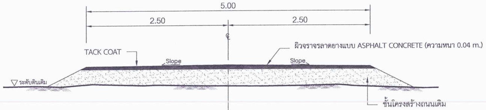
รูปตัดโครงสร้างทางแบบ ASPHALT CONCRETE NOT TO SCALE
