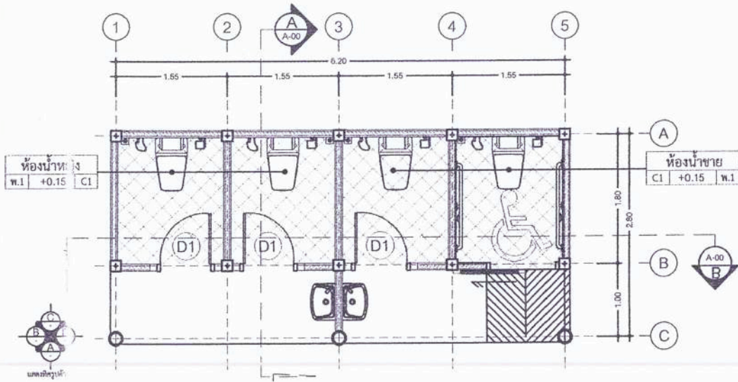
แปลนพื้นที่ห้องน้ำ มาตราส่วน 1:50
