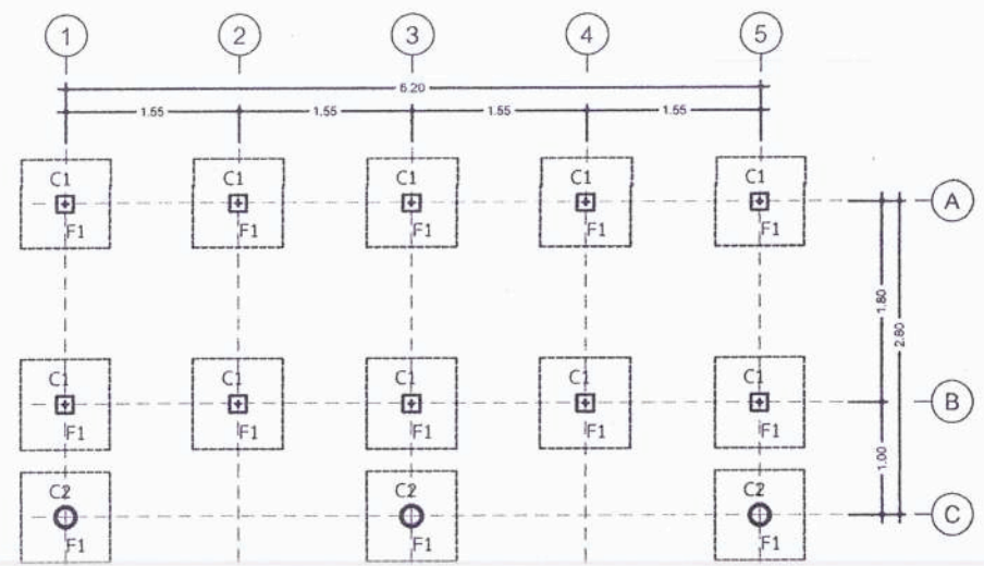
แปลนฐานราก มาตราส่วน 1:50
