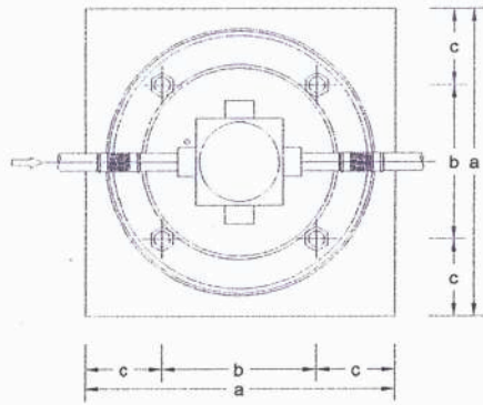
แปลน
