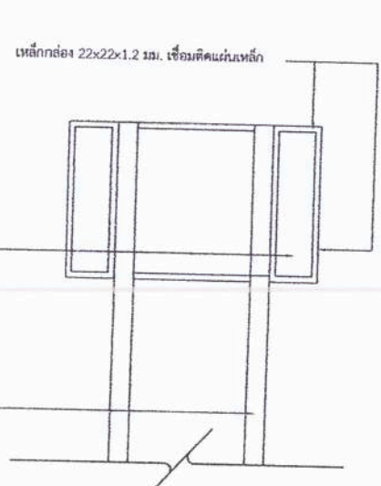
รูปด้านหลังแบบป้ายภายหลังการก่อสร้างเสร็จ
