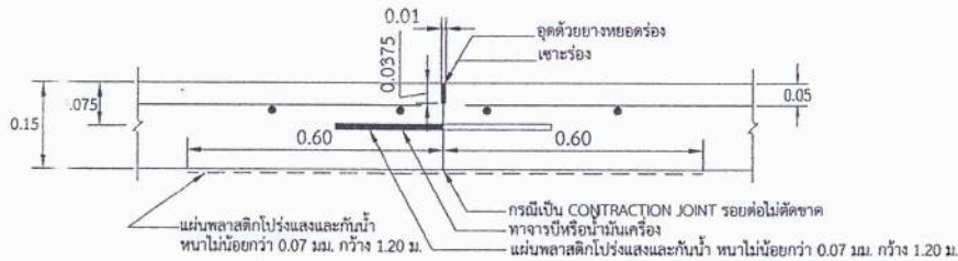
ขยายรอยต่อ CONTRACTION JOINT และ CONSTRUCTION JOINT
