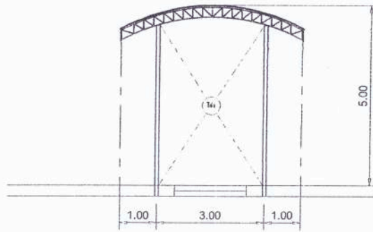
รูปด้านหน้าจุดปรับปรุง 1
