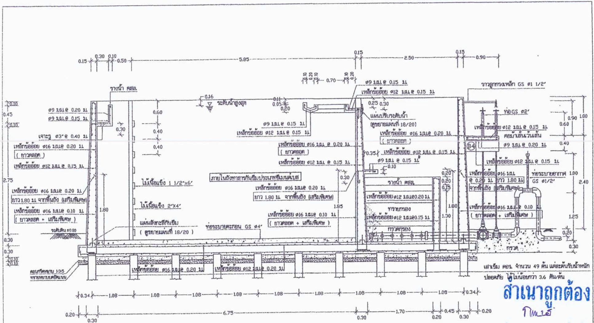
รูปตัด ๑ - ๑ 1:40
